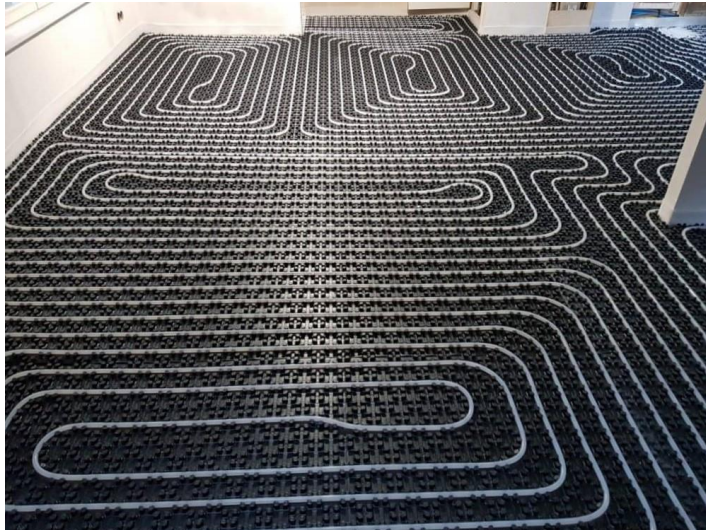
Vloerverwarming
